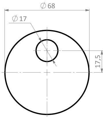
Draufsicht
