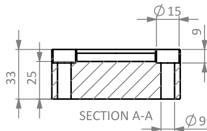
Obere Wippenstütze
